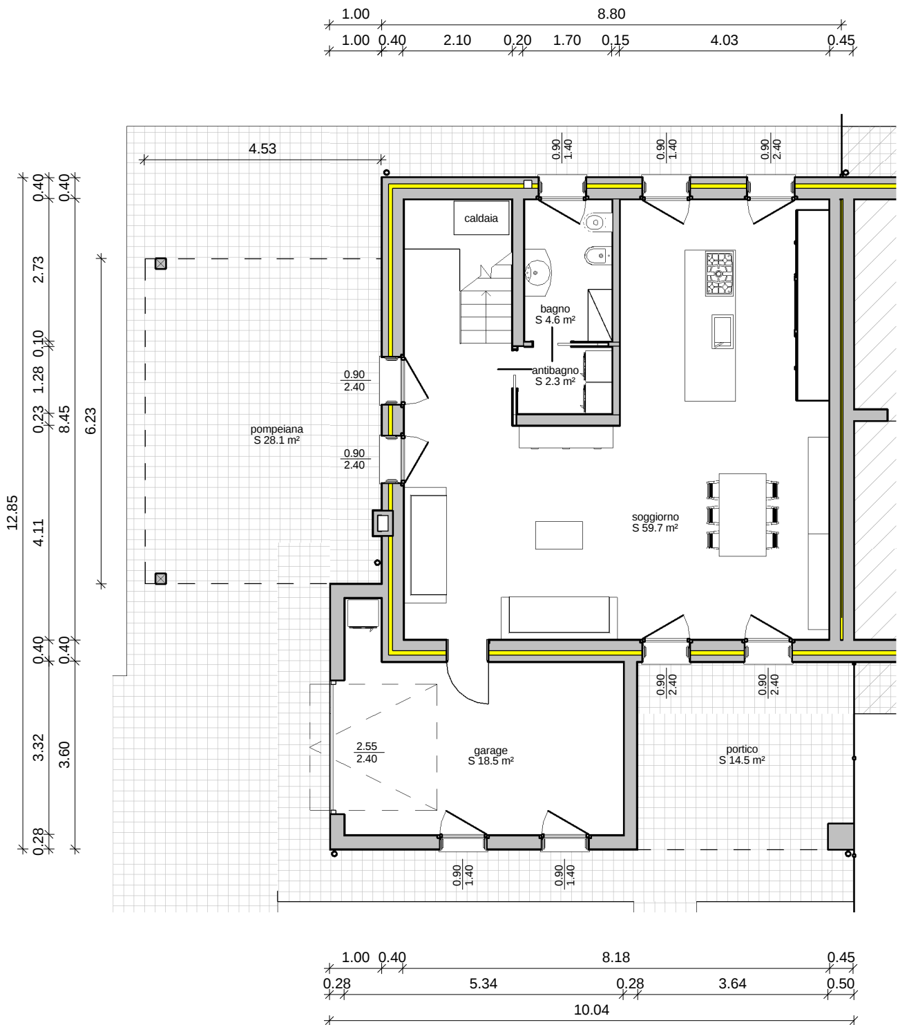
Unità A - Pianta piano terra
