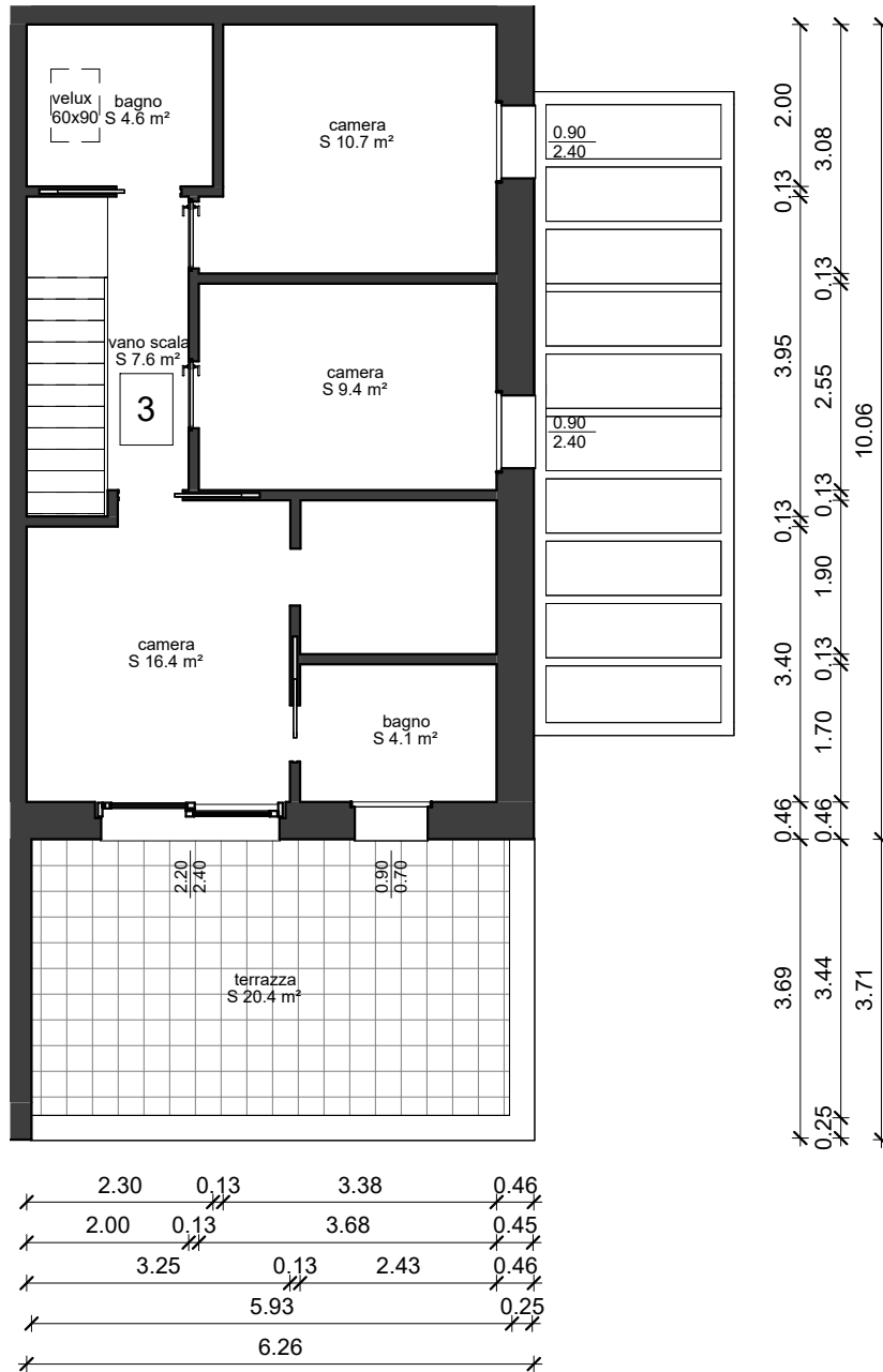
Piano primo 1:100
